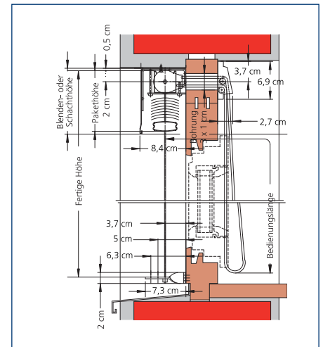
Typ Diplomat DA 50
