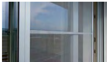
Schieberahmen (Option: mit Sprosse ohne Griffleiste)
